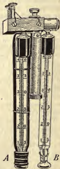
FIG. 3. Thermæsthesiometer.
